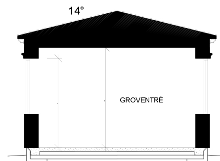
SEKTION B-B
