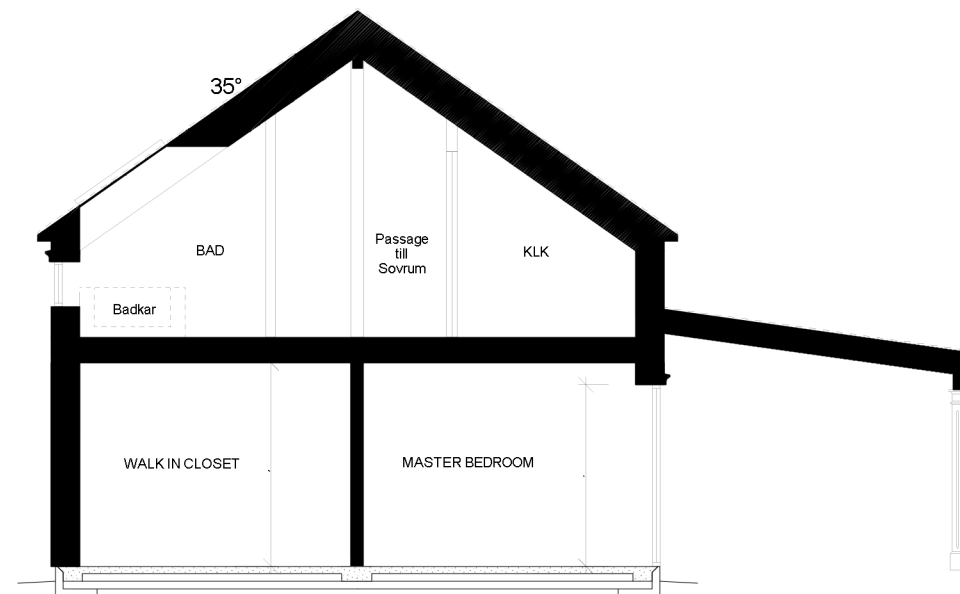
SEKTION C-C
